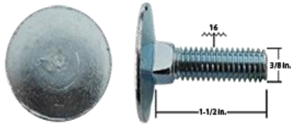
Tornillo para herraje de puerta 3/8" x 1 1/2" 16 hilos zincado
