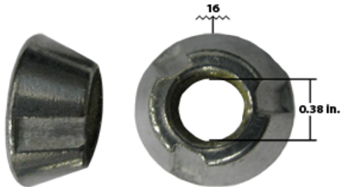
Tuerca de seguridad de 3/8, 16 hilos.
