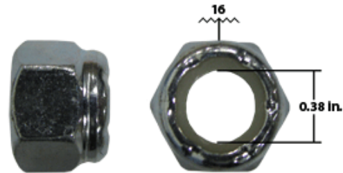
Tuerca hexagonal de 3/8", 16 hilos, con nylon.
